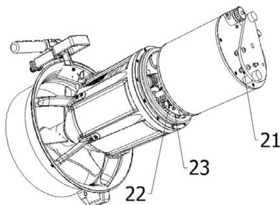
Figura 7 (vista dell'ADV senza l'involucro esterno)
